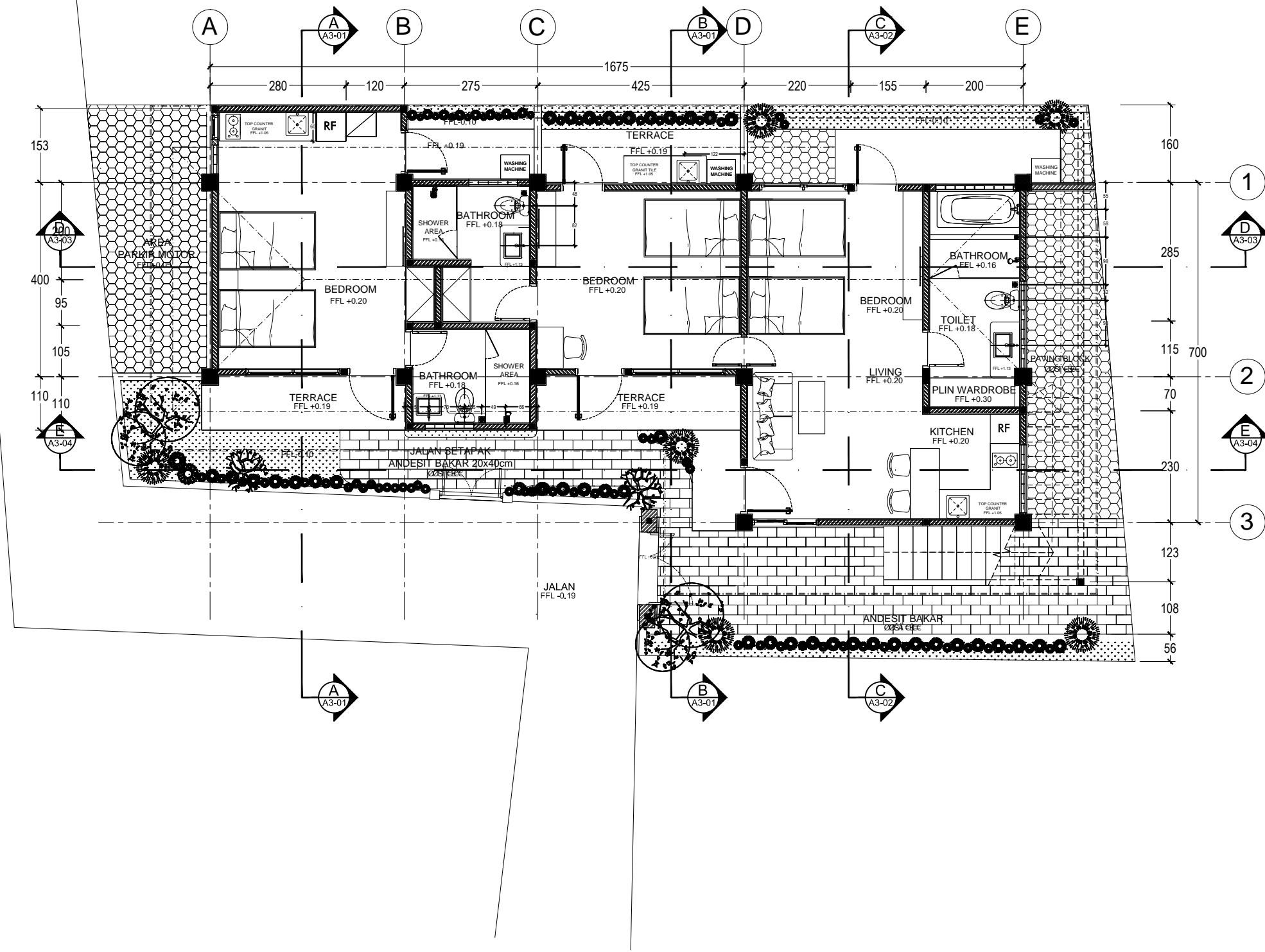
LAY OUT PLAN SKALA 1 : 100
